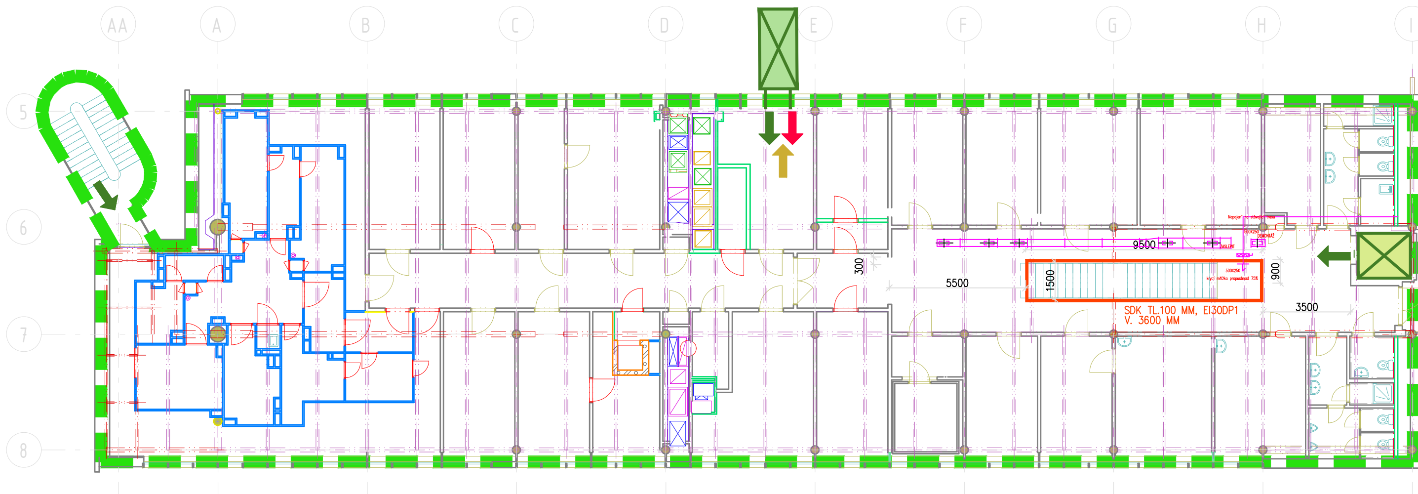
PŮDORYS 3.NP - FÁZE 2 - dočasná úprava stávajícího větrání CHUC
