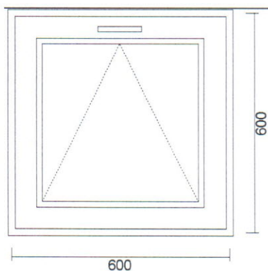
9. Okno 1- křídlové (pohled zevnitř)
