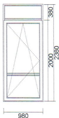
6. Okno 1- křídlové (pohled zevnitř)
