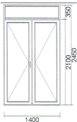
13. Dveře vnější (pohled zevnitř)
