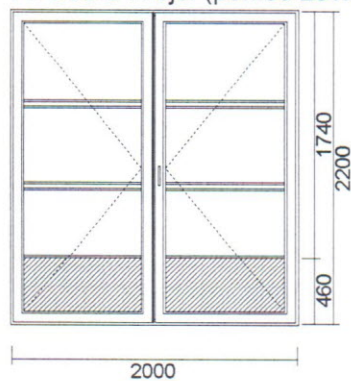
14. Dveře vnější (pohled zevnitř)
