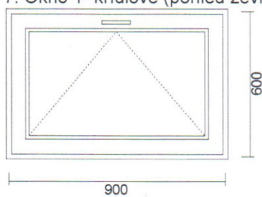
7. Okno 1- křídlové (pohled zevnitř)
