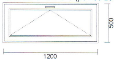
10. Okno 1- křídlové (pohled zevnitř)
