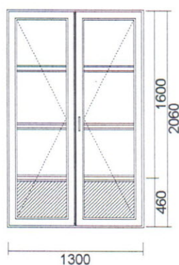
14. Dveře vnější (pohled zevnitř)
