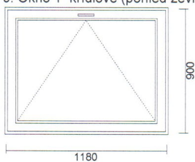
9. Okno 1- křídlové (pohled zevnitř)
