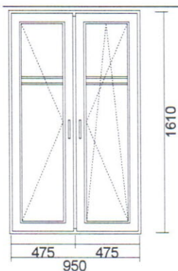
5. Balkonové dveře 1- křídlové (pohled zevnitř) 980 x 2380 mm
