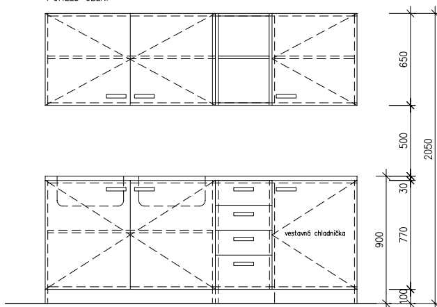
POHLED ČELNÍ
