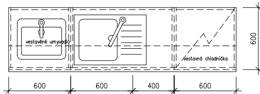
POHLED HORNÍ
