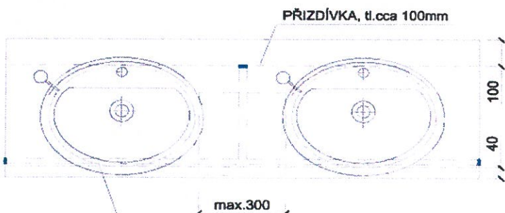
PŮDORYS
