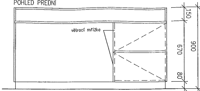
POHLED PŘEDNÍ
