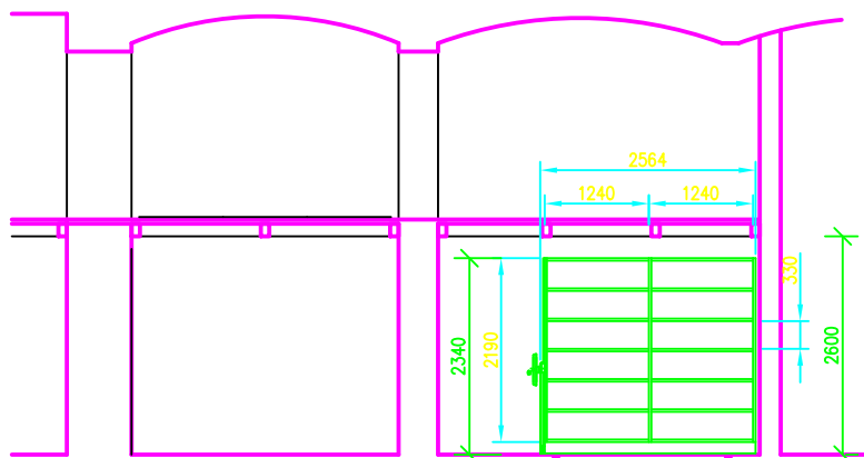
příčný řez
